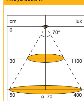
Diagramă de distribuție a luminii
