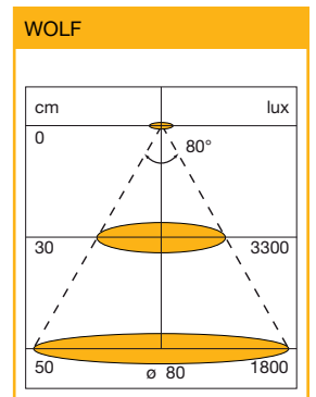
Diagramă de distribuție a luminii
