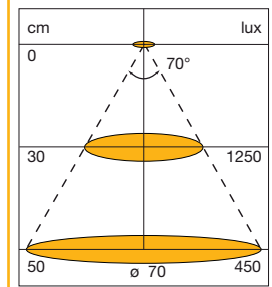
Diagramă de distribuție a luminii
