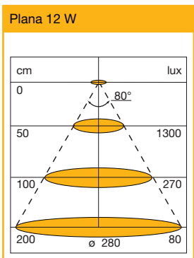
Diagramă de distribuție a luminii
