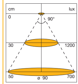
Diagramă de distribuție a luminii
