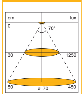
Diagramă de distribuție a luminii
