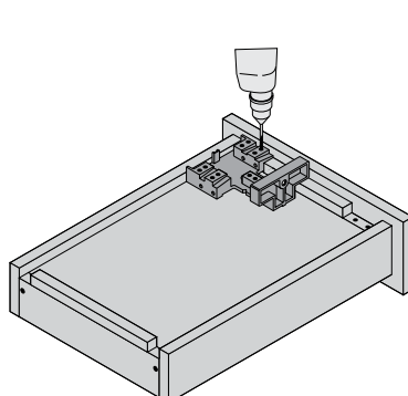
Prelucrare sertar – cuplaj Tandem
