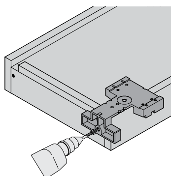
Prelucrare sertar – găurire sistem agățare
