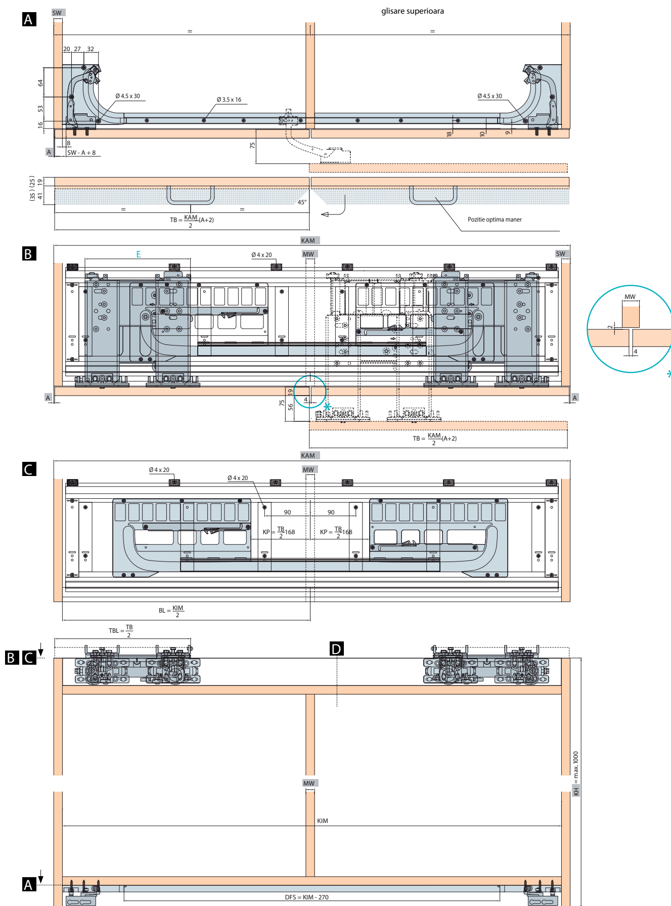
HAWA FRONTINO 20 H FS culisare superioară
