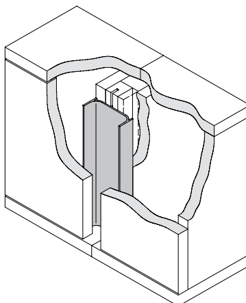
Profil în fața lateralelor de corp de mobilier
