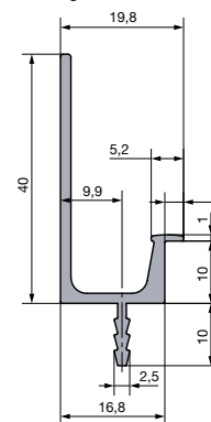
Profil maner Grande / Prego eloxat natur
