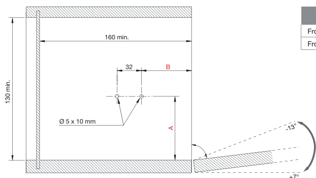
Bohrplan Korpusseite
