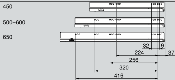
Pozitie insurubare sine corp – 70 kg
