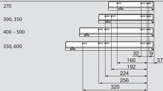
Pozitie insurubare sine corp – 70 kg
