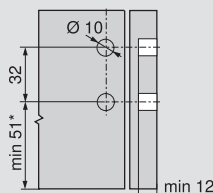
Cote de gaurire front, montare cu EXPANDO
