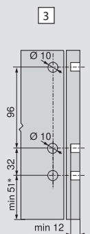
Cote de gaurire front, montare cu EXPANDO
