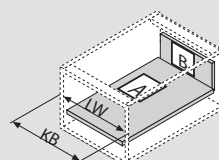
Cote debitare PAL 16 mm
