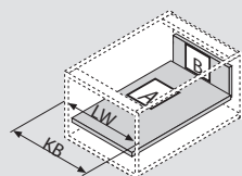
Cote debitare PAL 16 mm
