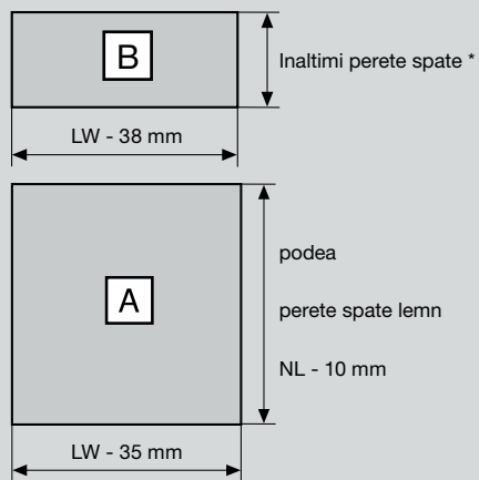
Cote debitare PAL 16 mm
