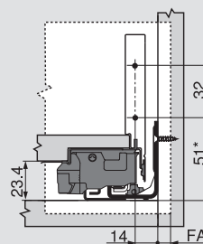
Cote de montare front cu suruburi
