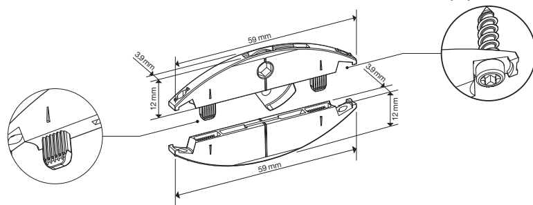
Grupa produs YL4
