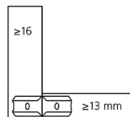
Imbinare prin forma
