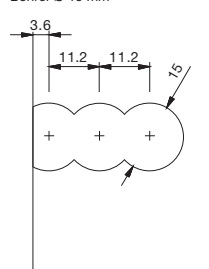
Schema de gaurire
